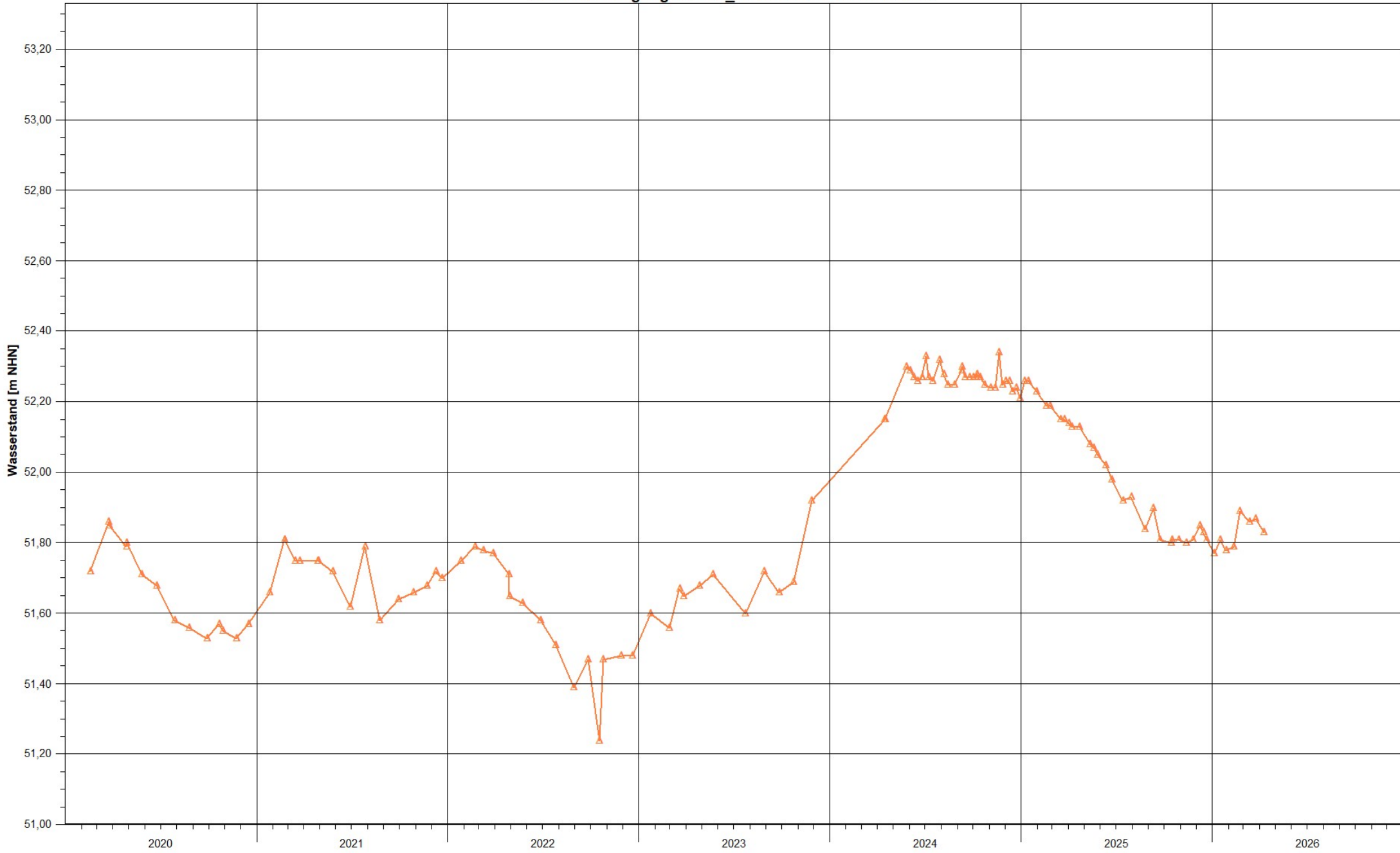
Grundwasserganglinie RS_47 01.01.2020 - 10.04.2026
