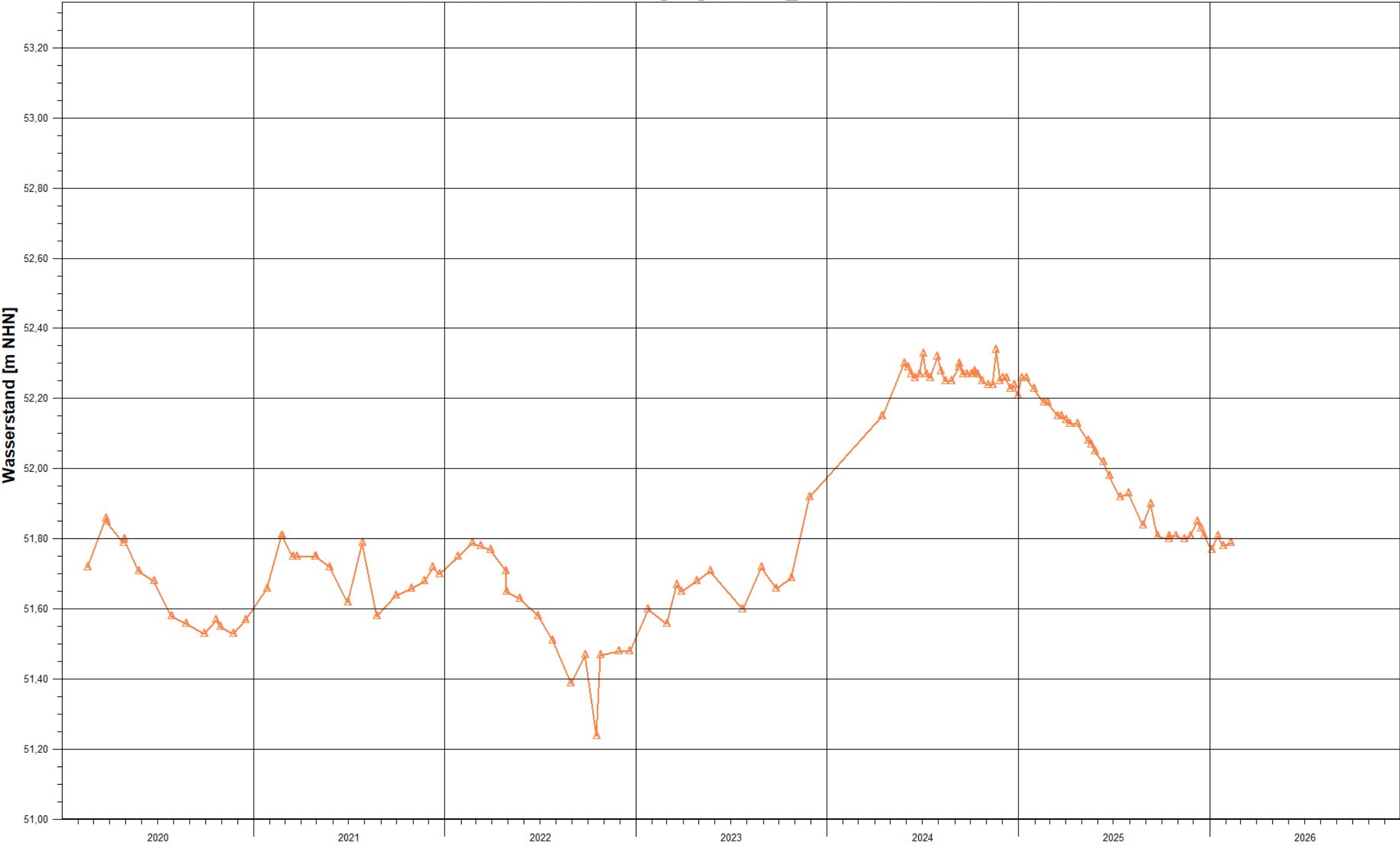
076748315, Grundwasserganglinie RS_47 01.01.2020 - 11.02.2026
